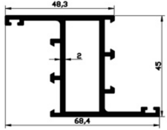
301.13 1,093 gr/mt
