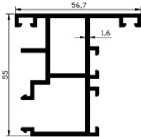
302.12 ADAPTÖR 1.087gr/m
