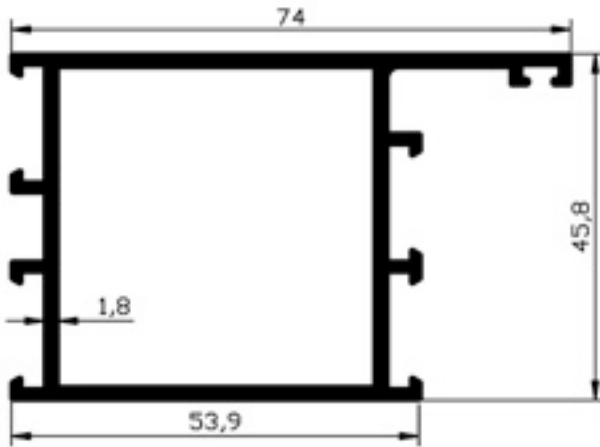
301.03 SİSTEM GENİŞ KASA 1.156gr/m
