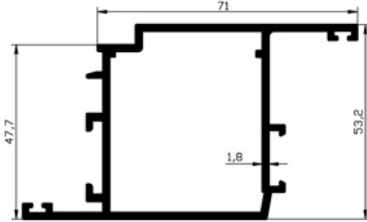
301.01 KANAT PROFİLİ 1.356gr/m
