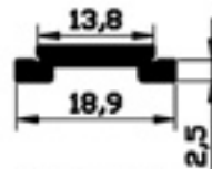
326.50 TİJ ÇUBUĞU 0.136 gr/m
