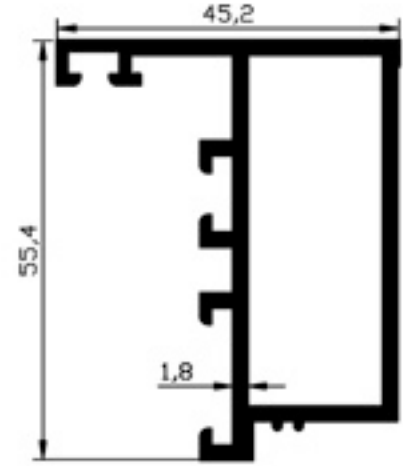
302.11 DAR KASA 0.969gr/m
