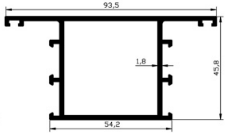
301.04 GENİŞ ÇİFT TIRNAK KASA 1.278gr/m
