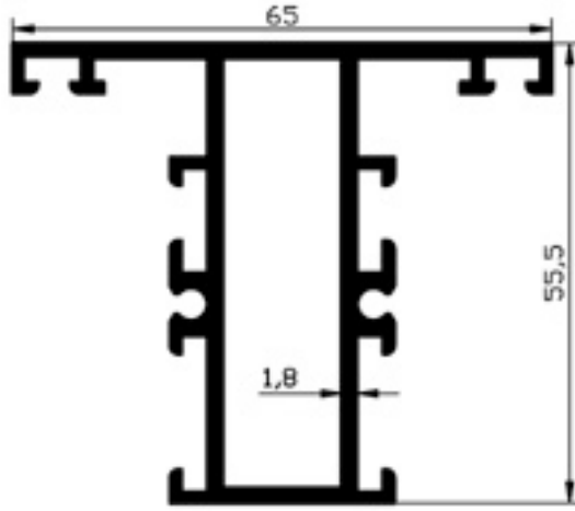
302.10 DAR ORTA KAYIT 1.228gr/m
