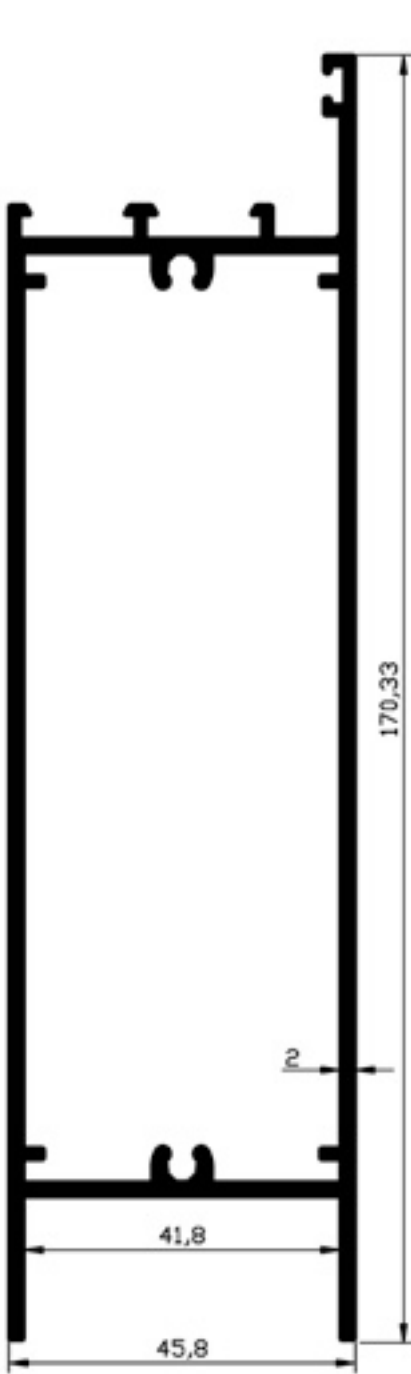
301.08 ALT BAZA 2.402gr/m
