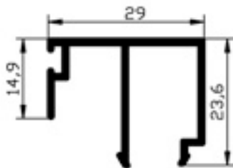
301.05 NORMAL CAM ÇİTASI 0.278gr/m
