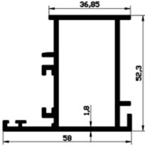
301.12 PİVOT ADAPTÖR 1,134 gr/mt
