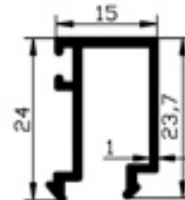
301.07 ISI CAM ÇİTASI 0.208gr/m
