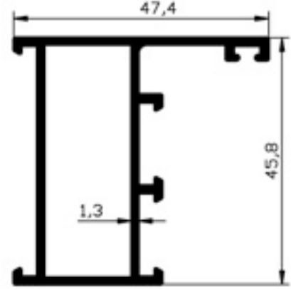
301.02 SİSTEM DAR KASA 0.671gr/m
